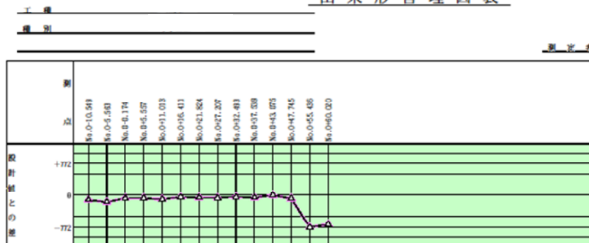
出来形管理図表
